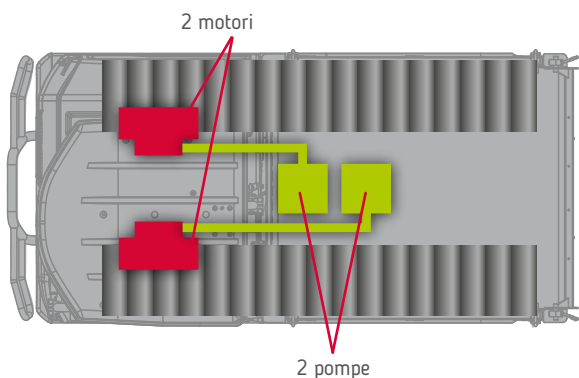
Sistema di trasmissione idrostatica HST (Hydrostatic System) a 2 pompe / 2 motori
